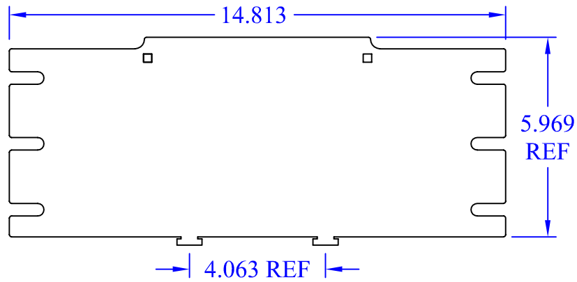
(1) WBT 6 IR
