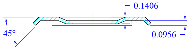
VIEW A-A
