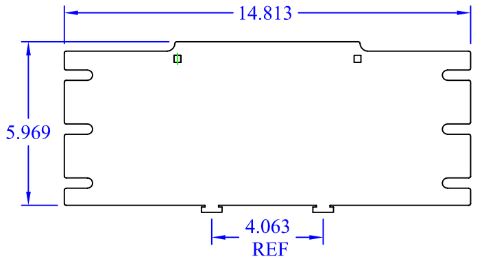
(2) WBT-6 IR
