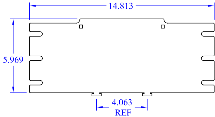
(2) WBT-6 IR
