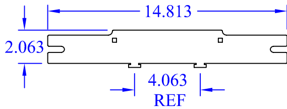
(4) WBT-2 IR
