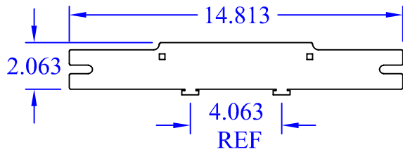
(4) WBT-2 IR
