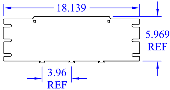
(1) WBT-45-6x8 OR
