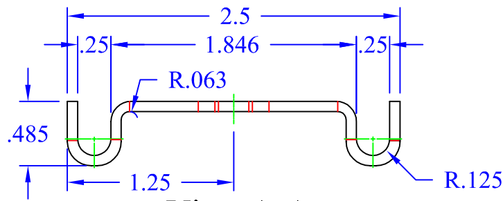
View A-A
