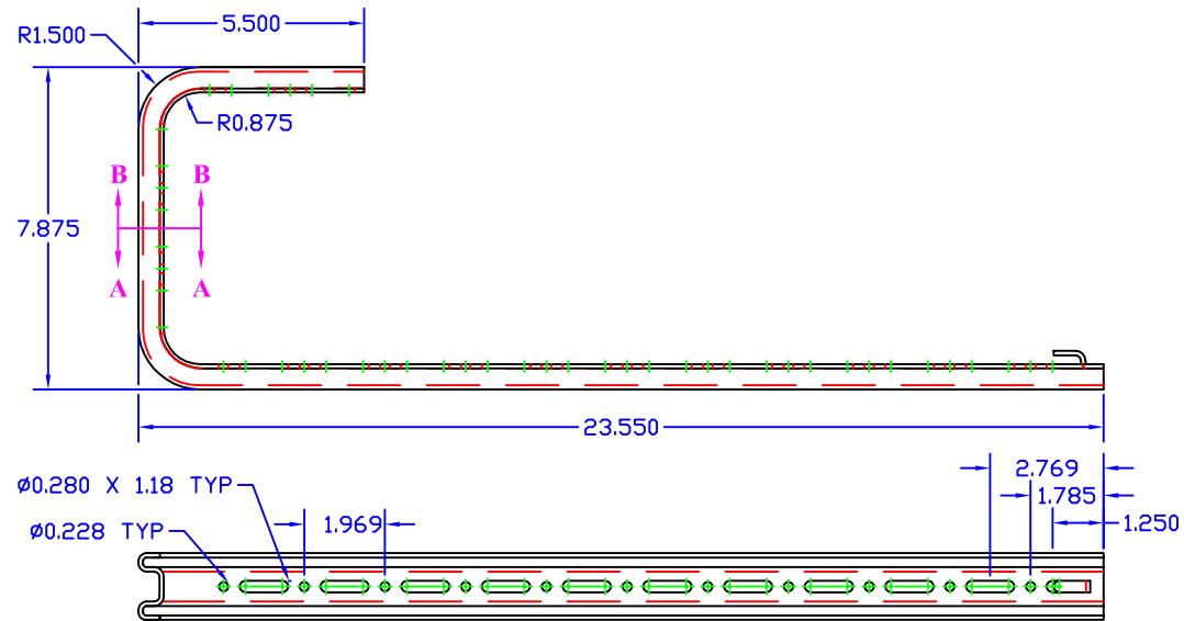
View A:A
